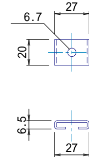
DNワッシャー詳細図 S=1:3
