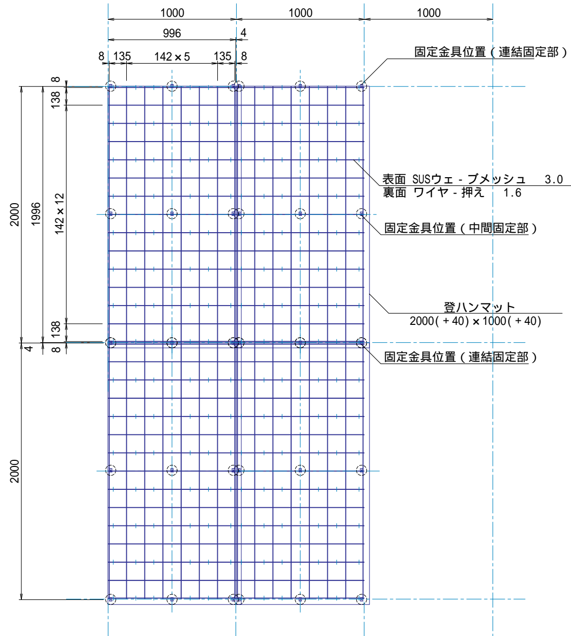
○ : 固定金具位置 正面図 (表面) S=1:30
