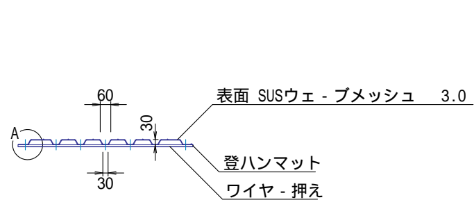
断面図 S=1:30
