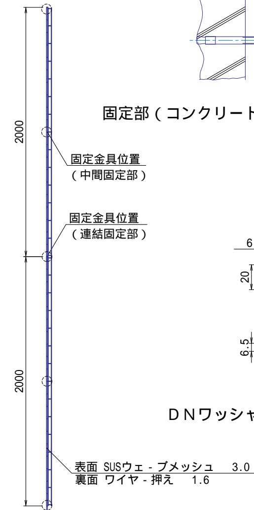
○ : 固定金具位置 側面図 S=1:30
