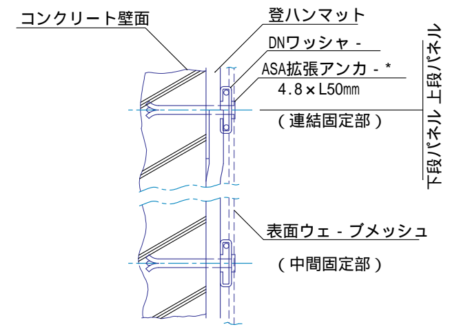
固定部 (コンクリート壁) 拡大断面図 S=1:3 * ツルパワーパネル本体の取り外しができない固定金具
