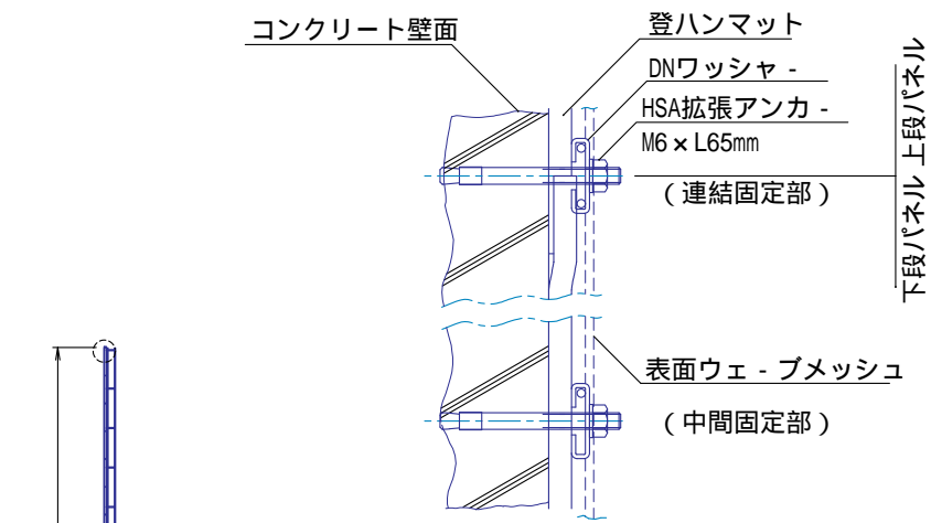
固定部 (コンクリート壁) 拡大断面図 S=1:3
