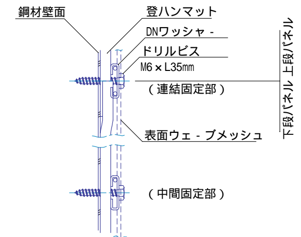
固定部 (鋼材壁面) 拡大断面図 S=1:3
