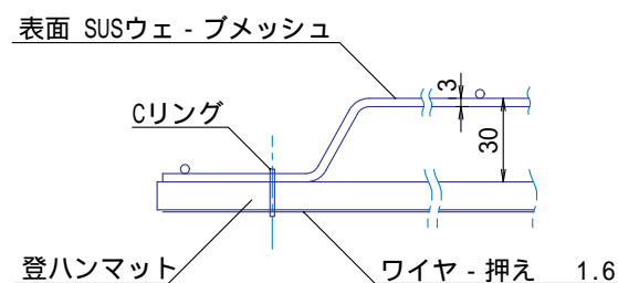
A部拡大断面図 S=1:3
