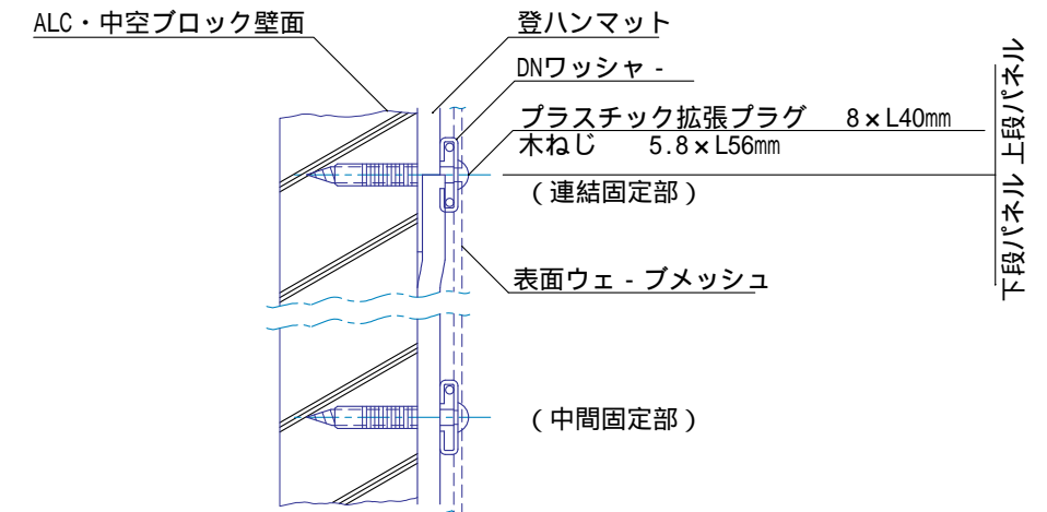
固定部 (ALC・中空ブロック壁) 拡大断面図 S=1:3
