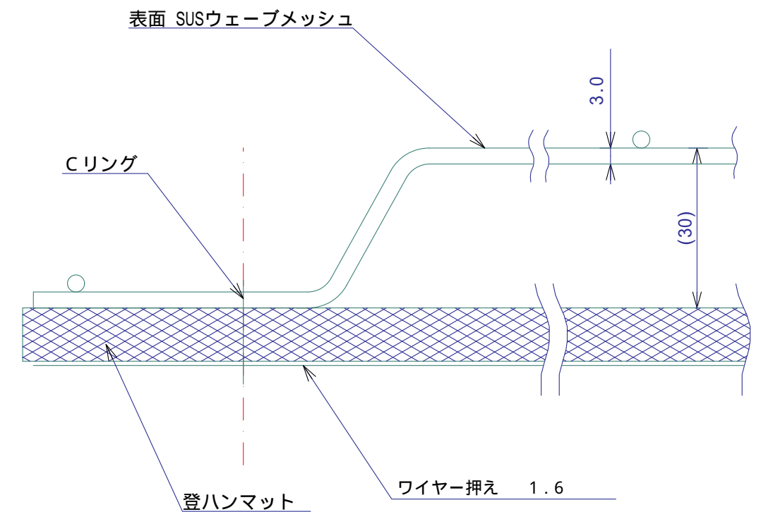
A部拡大断面図 S = 1 / 1
