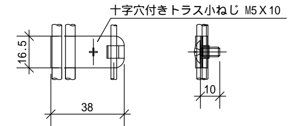
プランター連結金具詳細図 S=1/2
