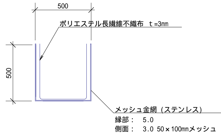
ツルメッシュプランター断面図
