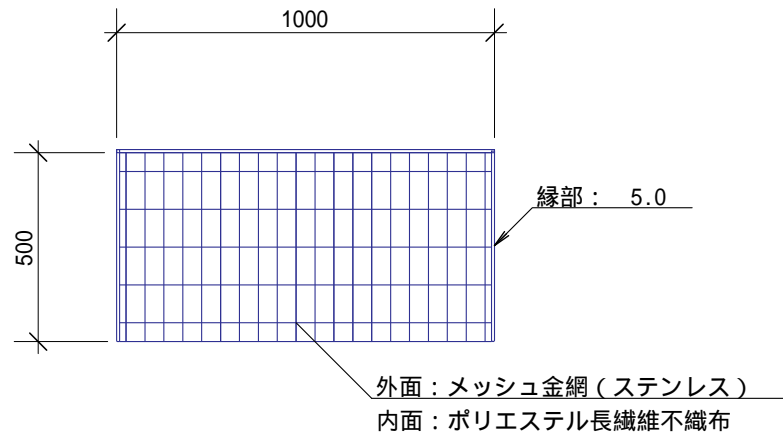
ツルメッシュプランター本体側面図
