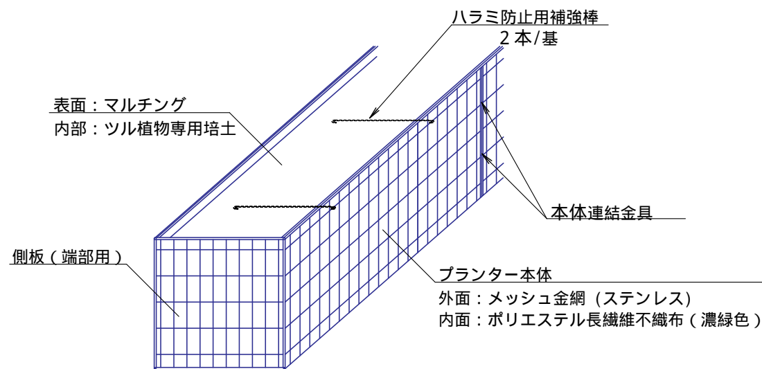
ツルメッシュプランター設置標準図
