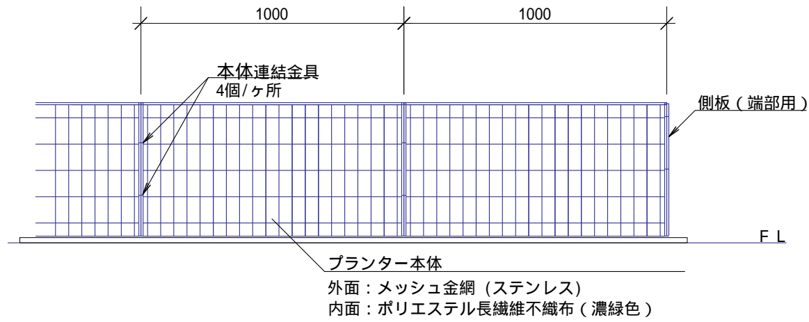
ツルメッシュプランター側面図
