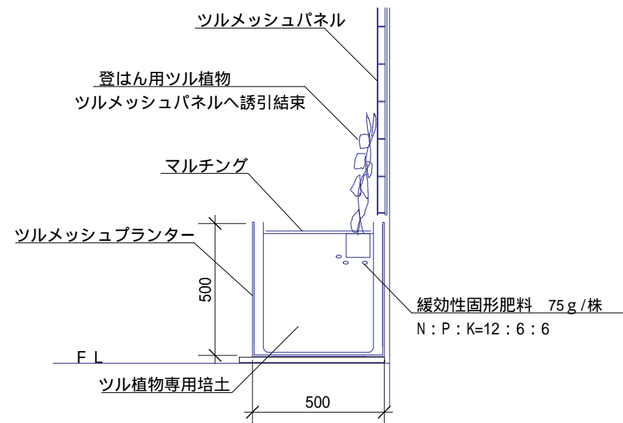
ツルメッシュプランター設置断面図
