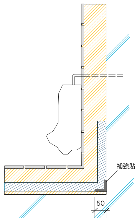
C部詳細図
