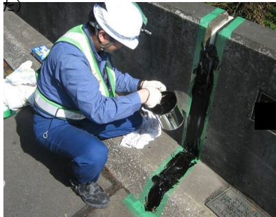
混合攪拌したスカイシール F-2 をゴムベラにて目地に充填。ベラにて平滑に仕上げる。
